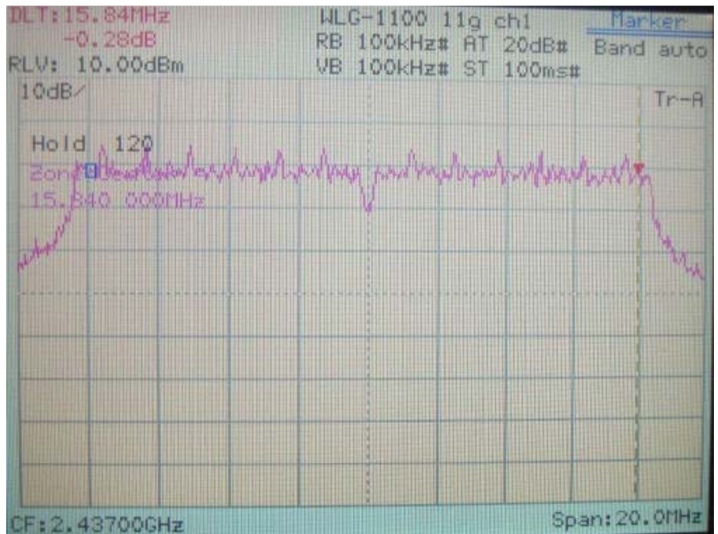
IEEE 802.11g
