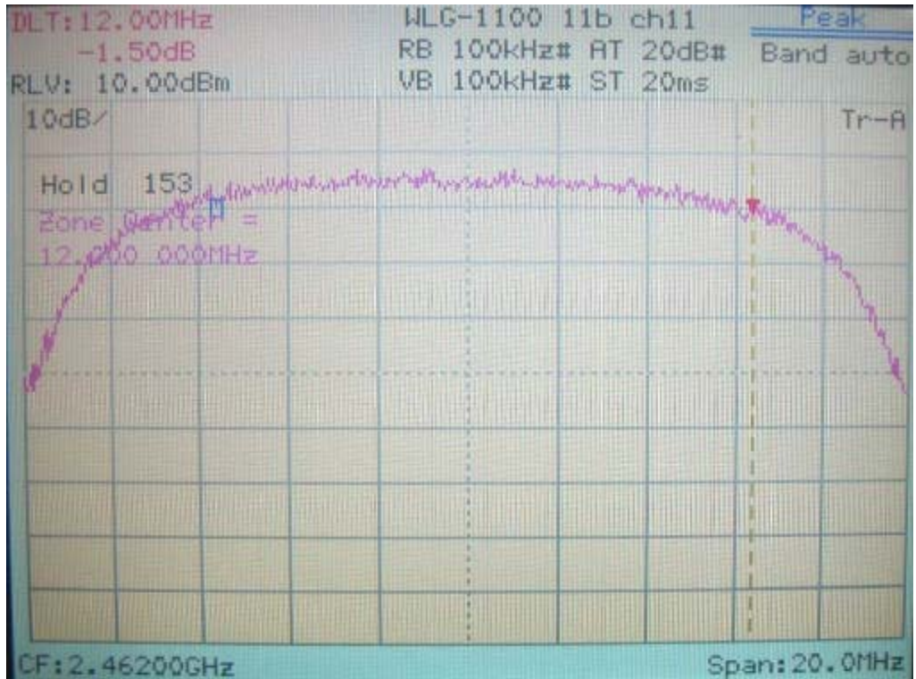
IEEE 802.11b
