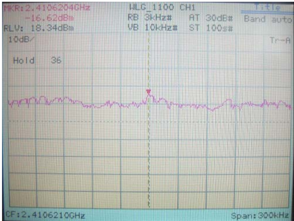
IEEE 802.11b
