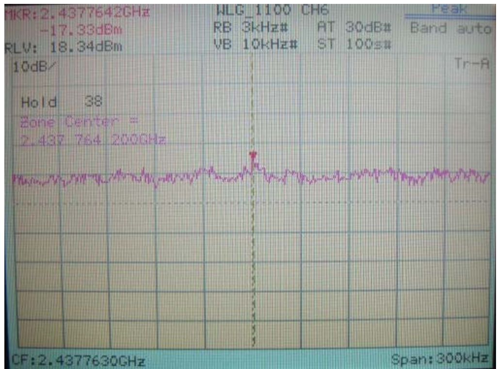
IEEE 802.11b
