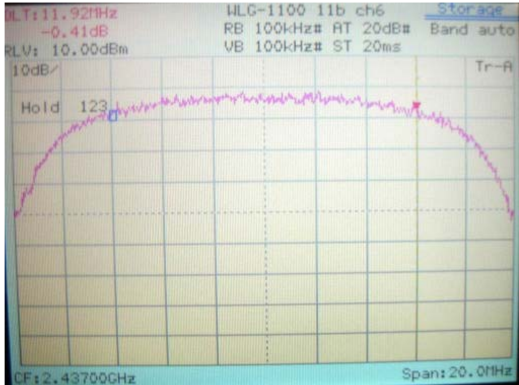
IEEE 802.11b
