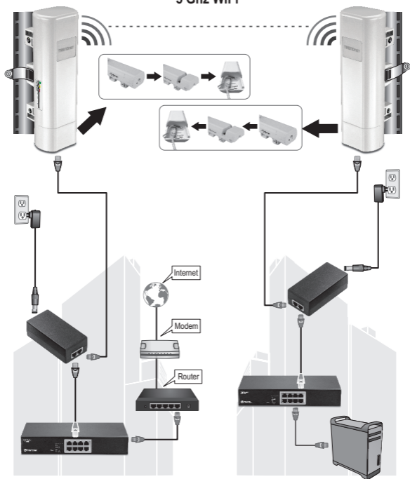
Edificio 1
