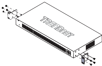
Fixation des supports sur le Switch
