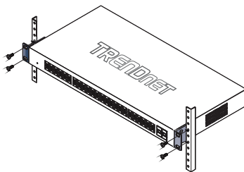
Installation du switch sur un rack
